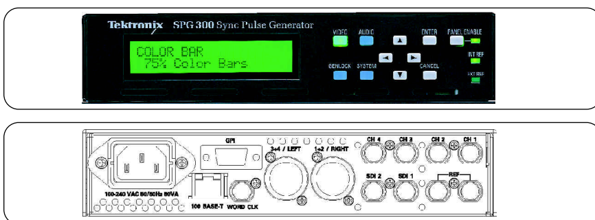
► SPG300(半机架宽)同步信号发生器的前后面板图示。
