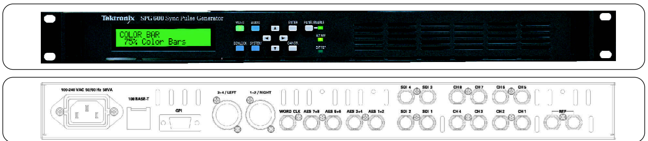
► SPG600(全机架宽)同步信号发生器的前后面板图示。
